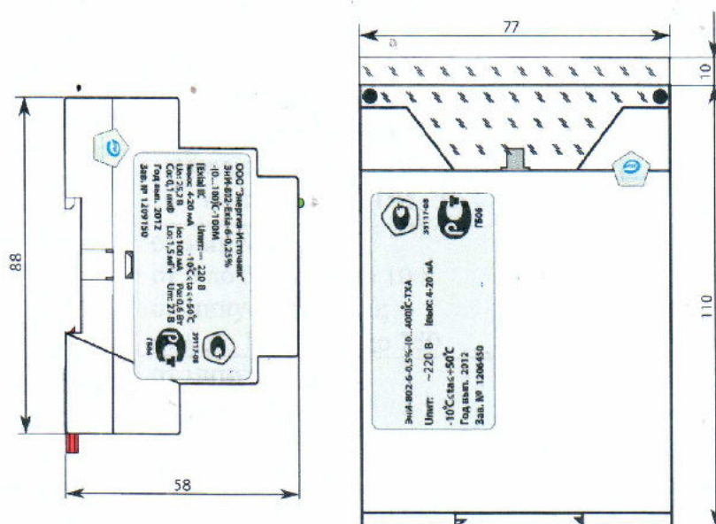
Рисунок 2 - Схема пломбировки ПИ
