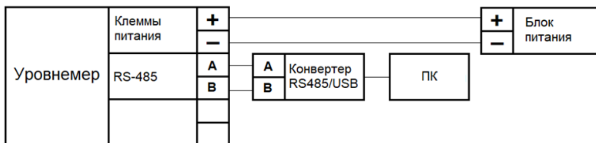
Рисунок Д.3 – Схема соединений уровнемера с кодом типа выходного сигнала М
