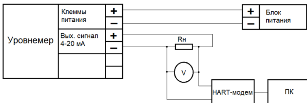
Рисунок Д.1 – Схема соединений уровнемера с кодом типа выходного сигнала Н
