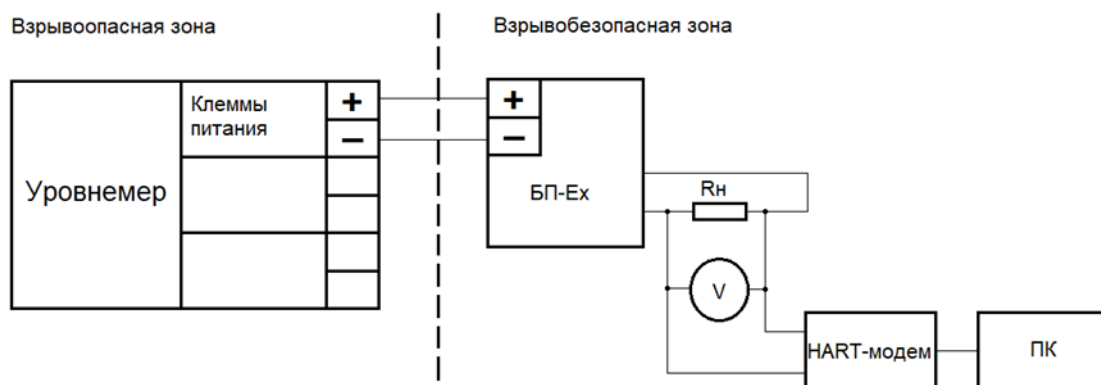
Рисунок Д.4 – Схема соединений уровнемера исполнения Exia с барьером искрозащиты с гальванической развязкой цепи питания и информационной цепи
