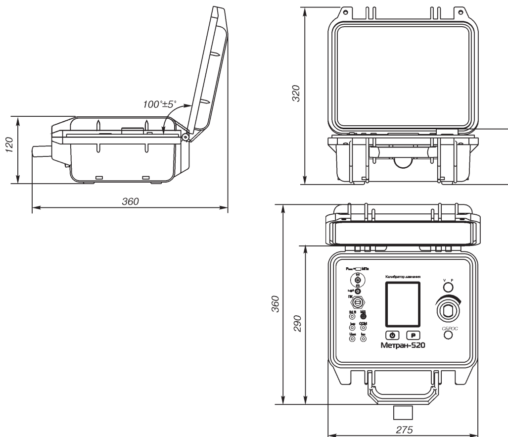
Рис. 5. Калибратор Метран-520-К.
