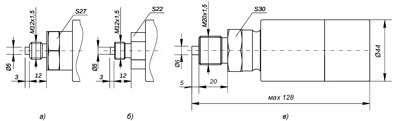
Рис. 4. Модуль давления общепромышленного исполнения.
