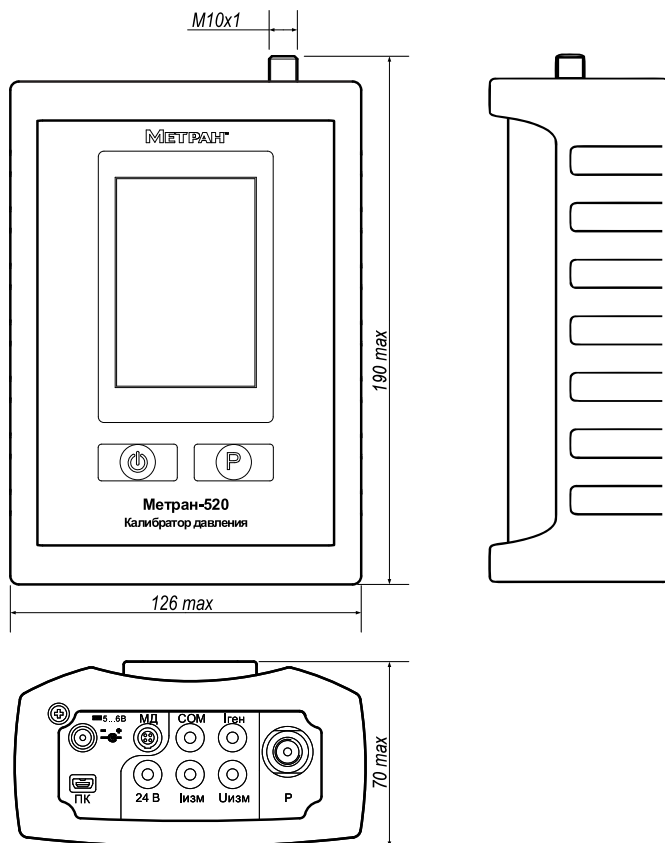
Рис.4. Калибратор Метран-520-Р.
