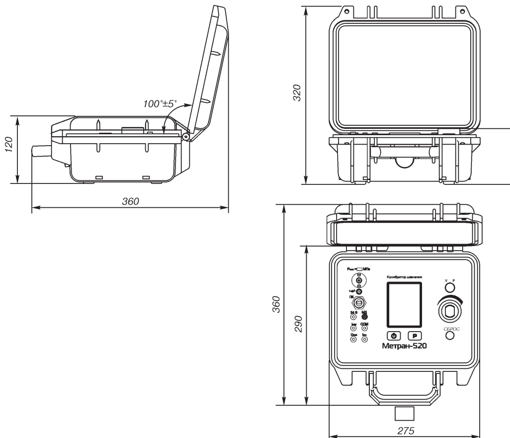
Рис.5. Калибратор Метран-520-К.
