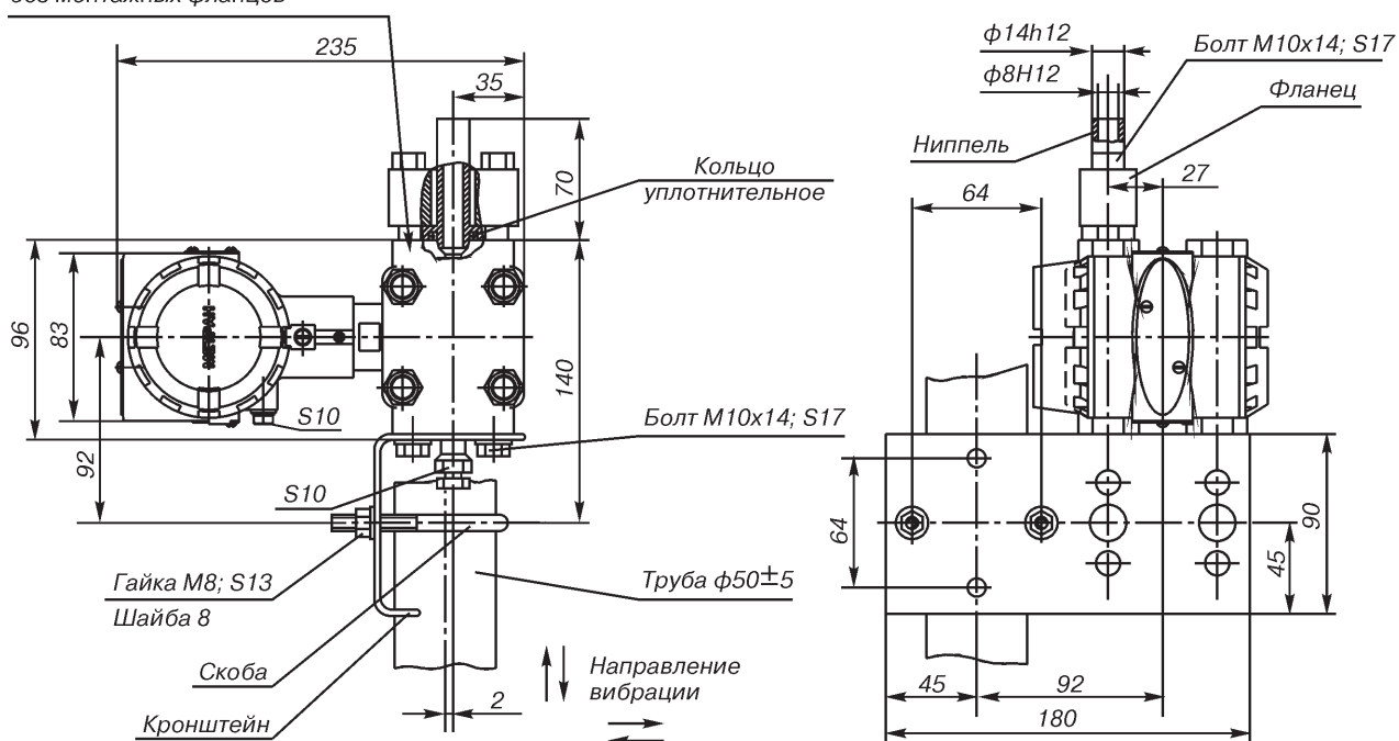
Рис.20. Датчики мод.150CG с установленным ниппелем (код D6) и монтажным кронштейном для установки на трубе с наружным диаметром до 50 мм (код B1).
