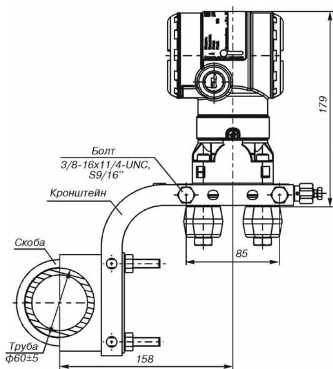
Рис.13. Датчики мод.150CDR и 150CGR с традиционным фланцем и монтажным кронштейном. Остальное см.рис.11.
