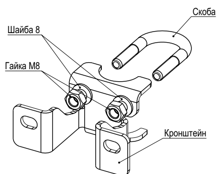
Рис.37 Кронштейн В1 или В4 для крепления на панели датчиков моделей 150TG и 150TA с кодами диапазонов 0T-5T
