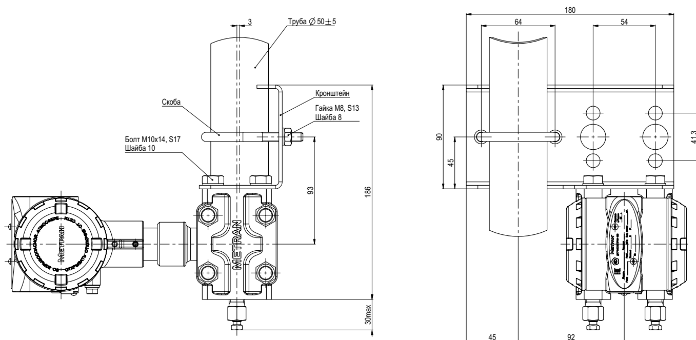
Рис.29. Датчики моделей 150CD, 150CG для кодов диапазона 1Т-5Т с монтажным кронштейном В1 или В4 (для установки на трубе или панели)
