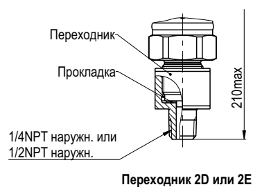
Рис.38. Датчики моделей 150TG, 150TA для кодов диапазона 0T-5T и кодом соединения с процессом 2G и переходниками.
