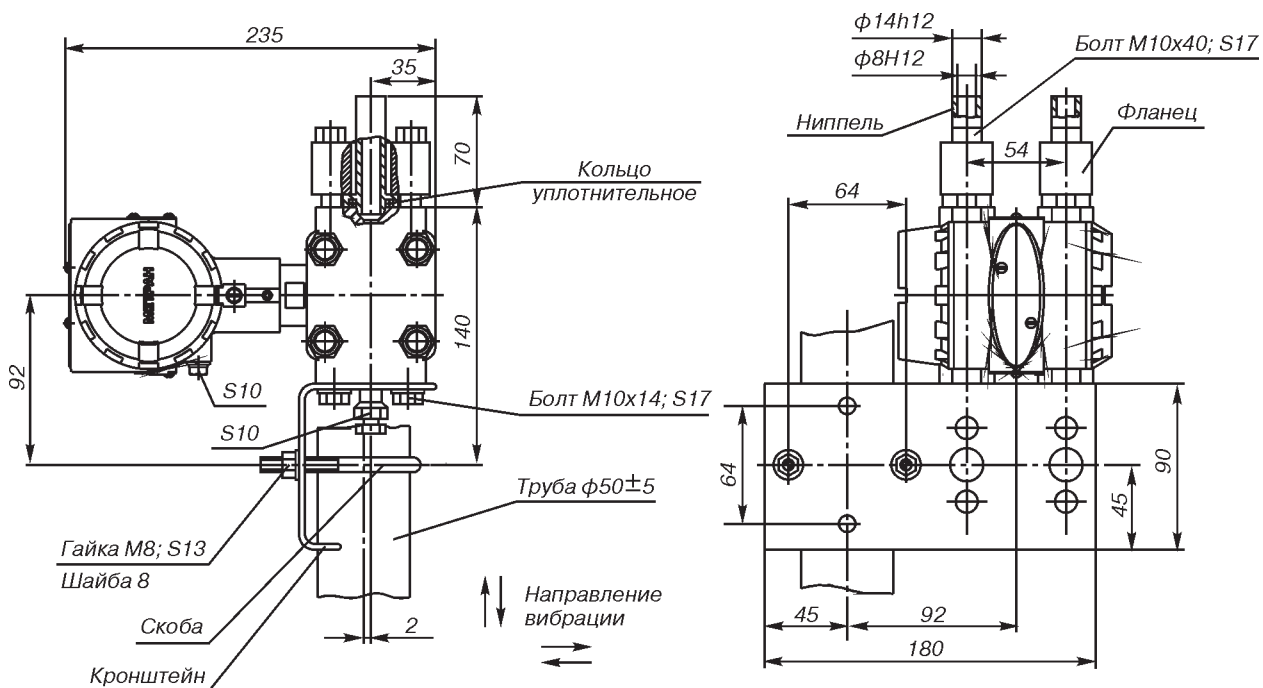
Рис.21. Датчики мод.150CD с установленными ниппелями (код D6) и монтажным кронштейном для установки на трубе с наружным диаметром до 50 мм (код B1).
