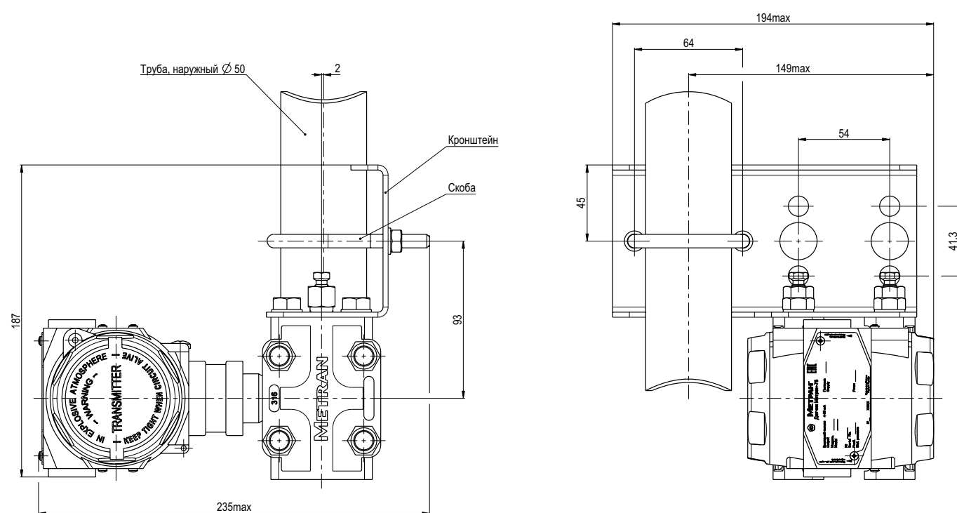
Рис.17. Датчики моделей 75CD/75CG с кронштейном В1 или В4
