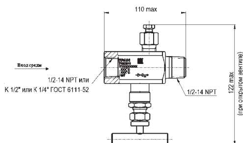
Рис.25. 1-вентильный блок модели 0106 М Т 1 с кодом соединения с процессом В (D) и типом соединения с датчиком А.
