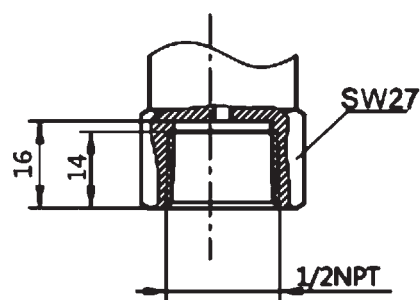
Рис.9. Датчики моделей 75TG/75TA с индикатором
