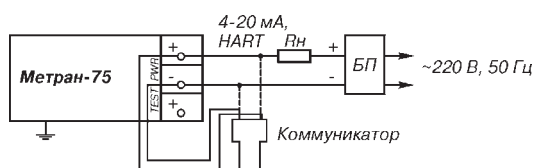
Рис.2. Выходной сигнал 4-20 мА (2-х-проводная линия связи).
