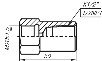
Рис.4. Переходник ПР3, ПР10.
