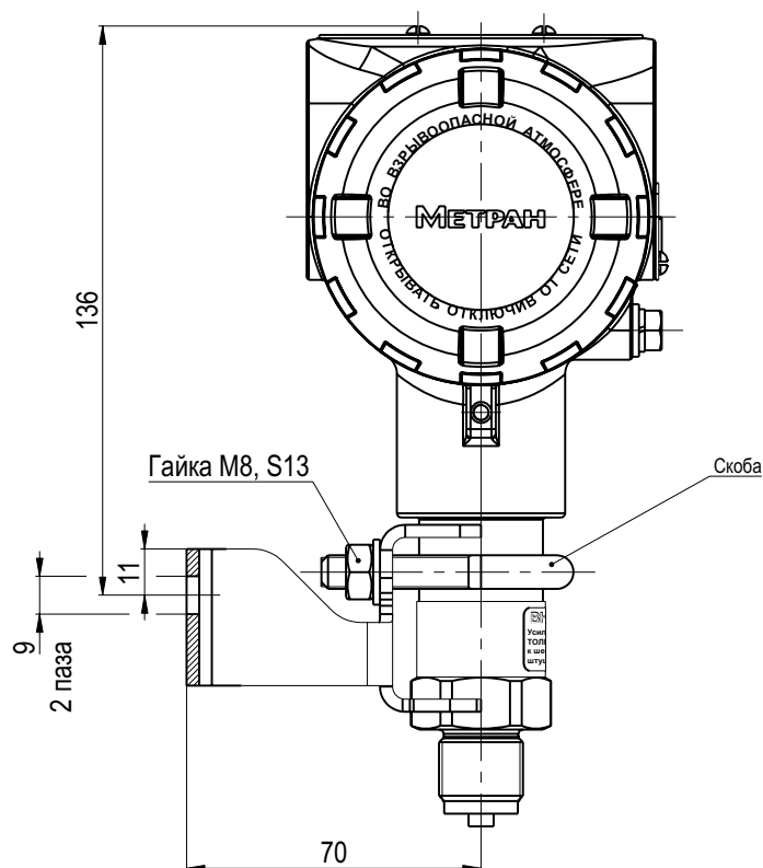
Рис.36. Датчики мод.150TG, 150TA для кодов диапазона 0T-5T и кодом соединения с процессом 2G и монтажным кронштейном В1 или В4 (для установки на панели)
