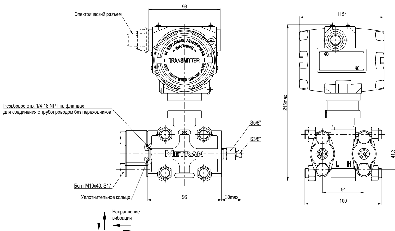
Рис.15. Датчики модели 75CD
