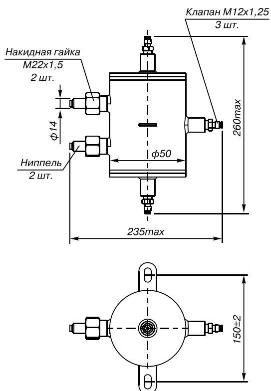
Рис.15. СР исполнения 04 (6,3; 25 МПа).
