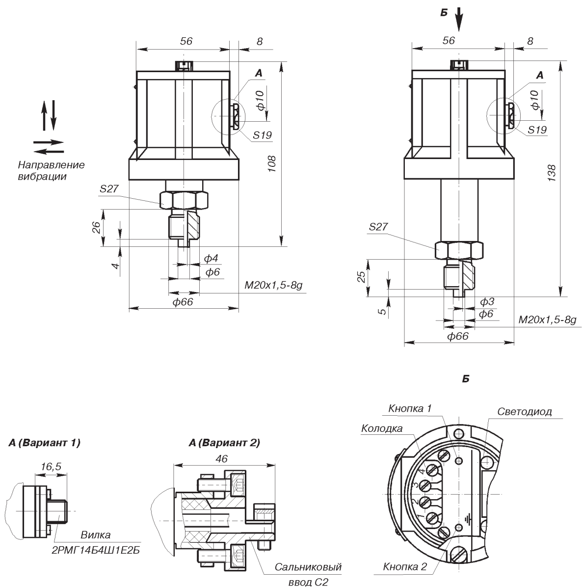
Рис.1. Метран-55, Метран-55-Ex, мод.515, 516, 517, 518, 528, 535.
