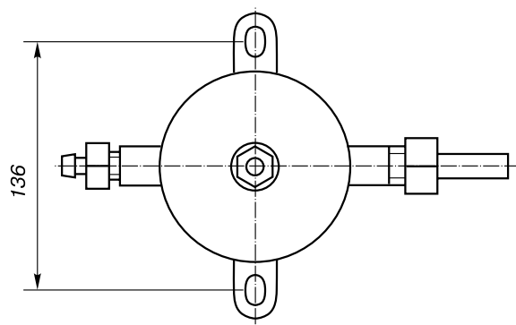
Рис.7. СР исполнения 4 (6,3; 25 МПа).
