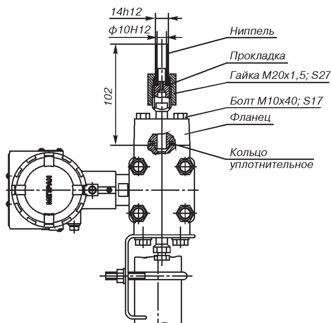
Рис.22. Датчики мод. 150CG с установленным ниппелем под накидную гайку M20x1,5 (код D5) и монтажным кронштейном для установки на трубе с наружным диаметром до 50 мм (код B1).
