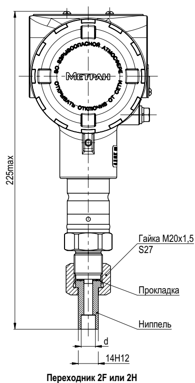
Рис.38. Датчики моделей 150TG, 150TA для кодов диапазона 0T-5T и кодом соединения с процессом 2G и переходниками.
