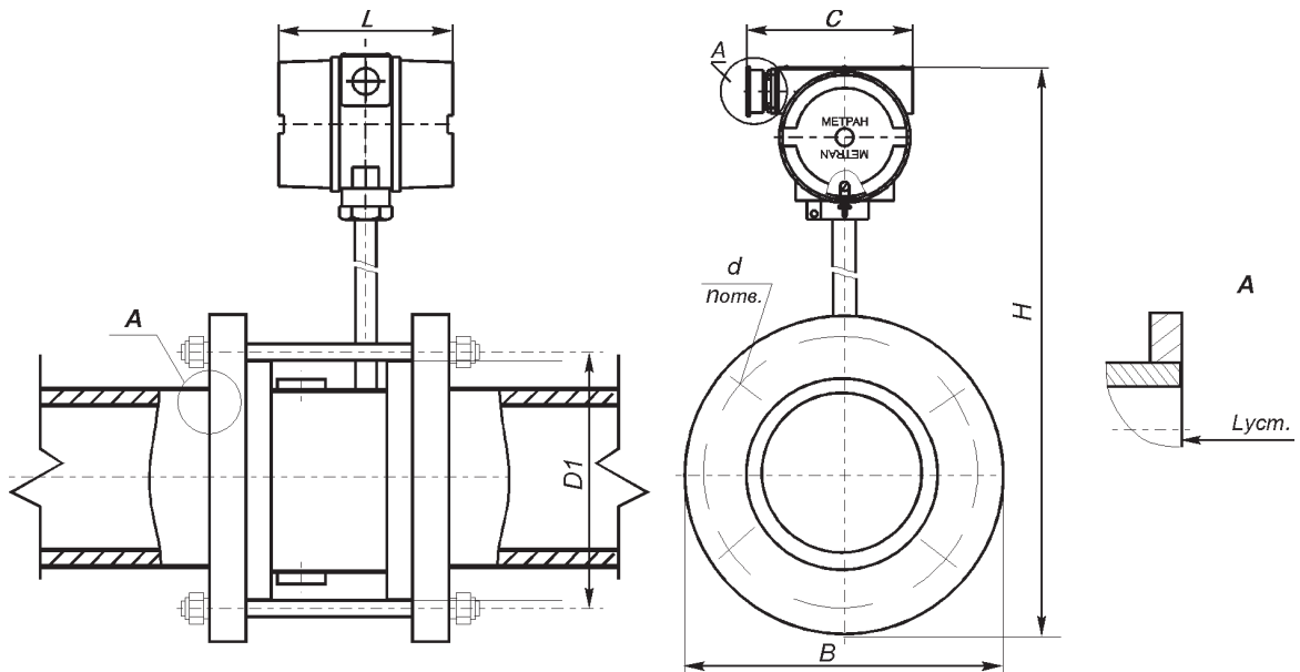
Рис.8. Расходомер Метран-300ПР, Ду 250, 300; с подключением через штепсельный разъем (код "ШР2").
