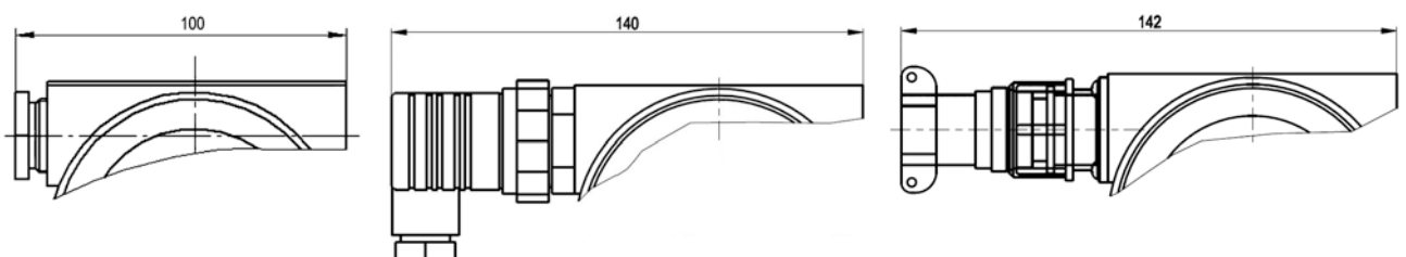
Рис.10. Подключение через сальниковый ввод (код "С"), через штепсельный разъем с установленной розеткой типа 2РМГ22КПН10Г1В1 (код "ШР") и через разъем DIN 43650а (код "Д")
