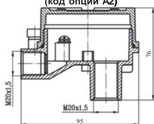
Соединительная головка (код опции A2)
