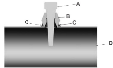
Рис. 2. Компоненты резьбового монтажа
