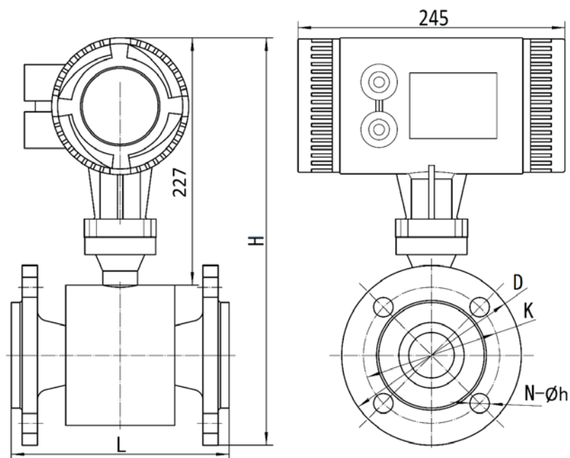
Рис. 16. Расходомер модели Метран-370MR с преобразователем интегрального монтажа.
