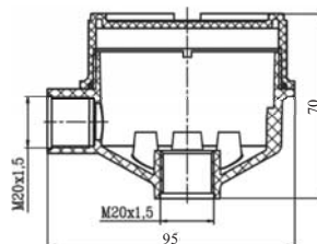
Соединительная головка (код опции P1)
