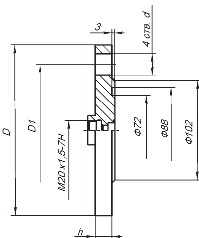
Рис. 9. Фланец гильзы 2004-05; 2004-15. Исполнение D; DN 50, PN: 10...200
