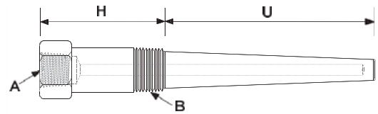
Коническая резьба
