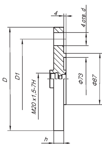
Рис. 8. Фланец гильзы 2004-04; 2004-14. Исполнение С; DN 50, PN: 10...200
