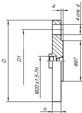
Рис. 6. Фланец гильзы 2004-02; 2004-12. Исполнение Е; DN 50, PN: 10...200
