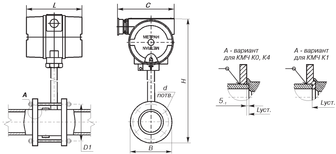
Рис.7. Расходомер Метран-300ПР-А (Ду25...100); с подключением через штепсельный разъем (код "ШР2").
