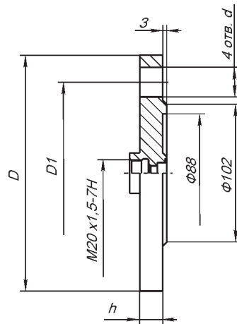
Рис. 7. Фланец гильзы 2004-03; 2004-13. Исполнение F; DN 50, PN: 10...200
