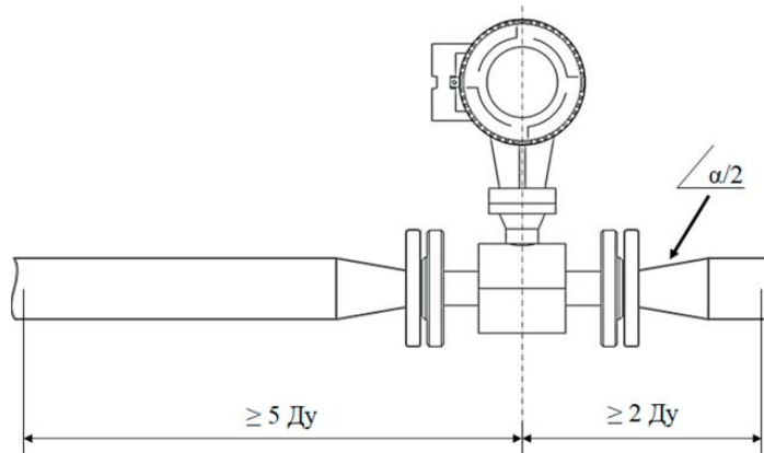
Рис. 13. Требование прямых участков при применении монтажного комплекта со встроенными коническими переходами.
