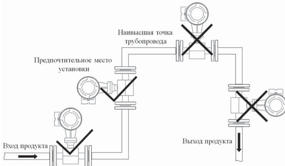
Рис. 11. Предпочтительное место установки расходомера.
